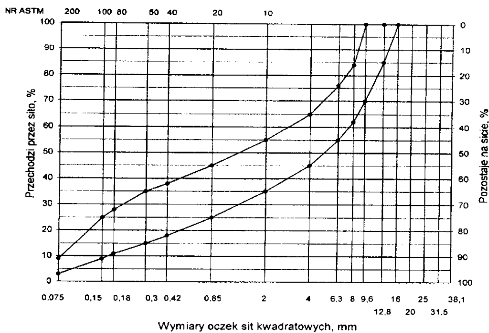
Rys. 9. Krzywe graniczne uziarnienia mieszanki mineralnej BA od 0 do 16 mm do warstwy wiążącej, wyrównawczej i wzmacniającej nawierzchni drogi o obciążeniu ruchem KRI lub KR2
