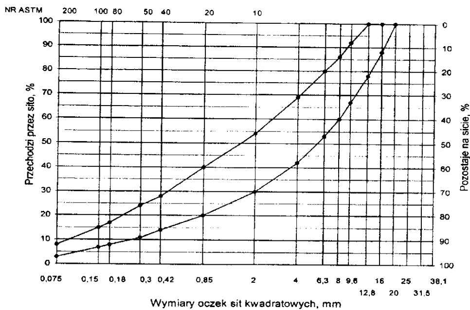
Rys. 8. Krzywe graniczne uziarnienia mieszanki mineralnej BA od 0 do 20 mm do warstwy wiążącej, wyrównawczej i wzmacniającej nawierzchni drogi o obciążeniu ruchem KRI lub KR2
